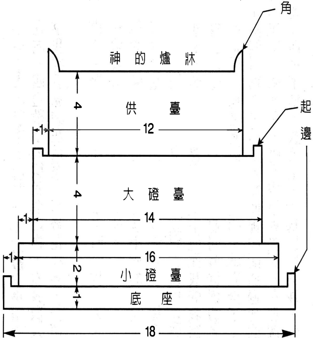
第三圖：祭壇尺寸圖(四三13~17)
